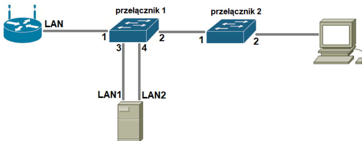
Schemat połączeń urządzeń w sieci lokalnej
